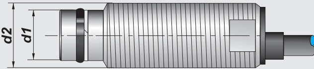
Схема монтажная №1
